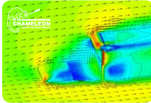
Simulación de la desviación del aire con un software de análisis de flujo.
